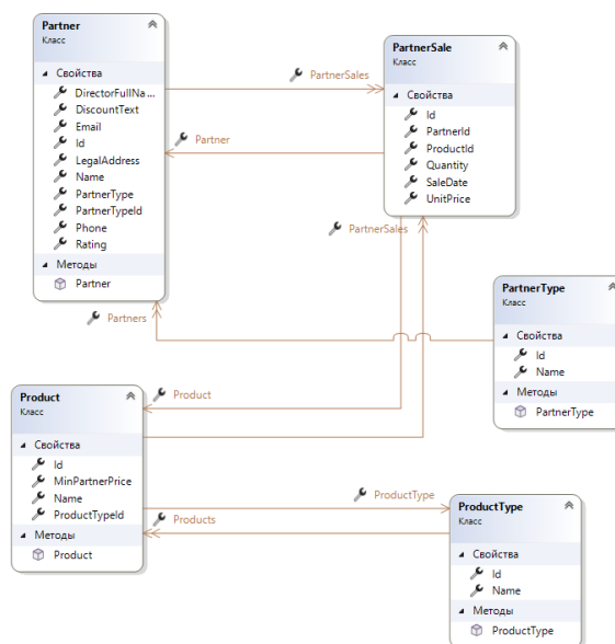
Рисунок 2.1.4 -Диаграмма классов
